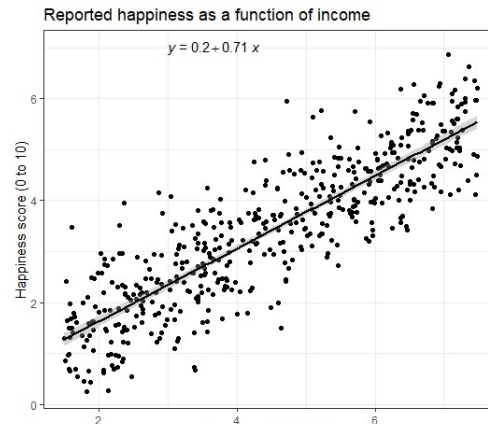
Linear Models
